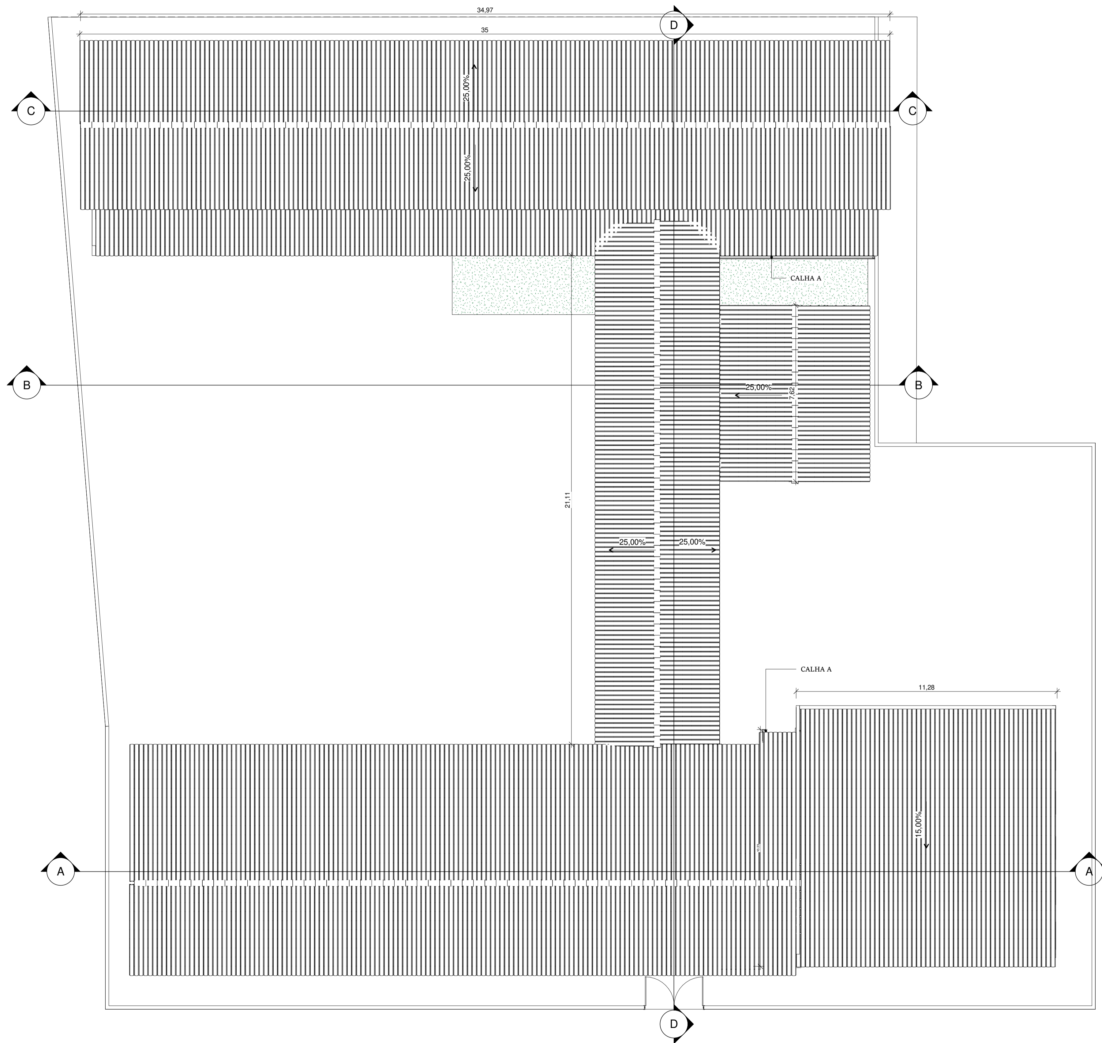
7 DIAGRAMA DE COBERTURA E LOCAÇÃO ESCALA 1 : 100
