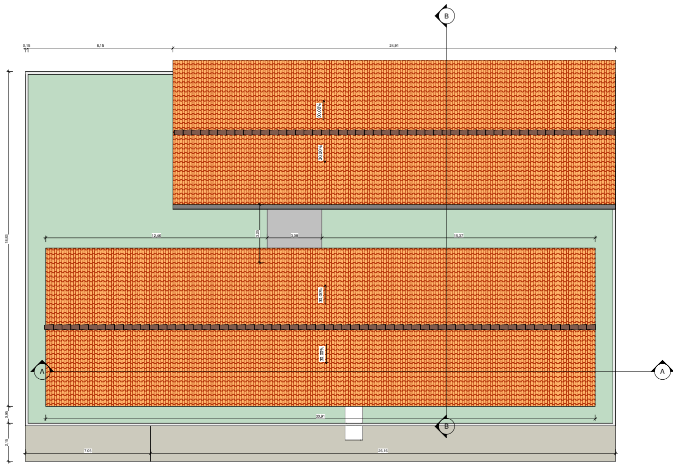
9 PLANTA DE COBERTURA E LOCAÇÃO ESCALA 1:75
